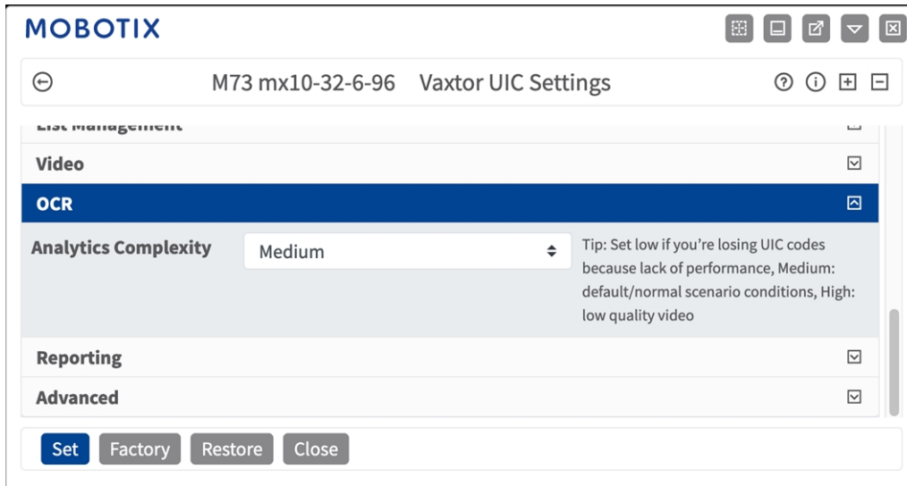
Fig. 9: OCR
