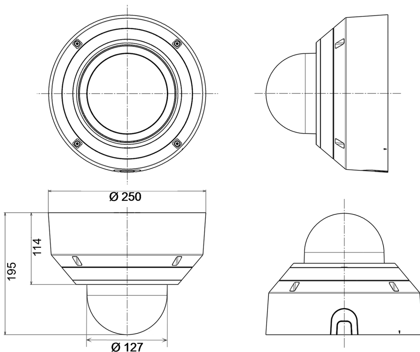
Abb. 1: Mx-VMSD1A-2021-VA: Alle Maße in mm
