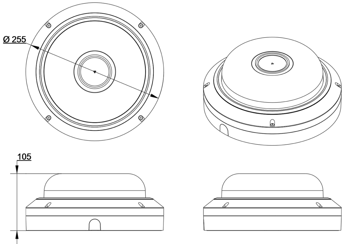
Fig. 1: Mx-VM1A-20-IR-VA: Todas las medidas en mm
