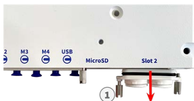
Fig. 5: Retire la cubierta de la ranura de la tarjeta de interfaz
