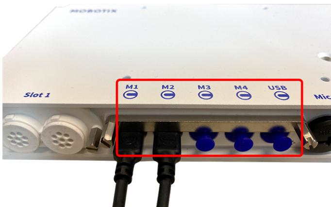
Abb. 4: 4 Modulsteckeranschlüsse und 1 USB-C-Schnittstelle
