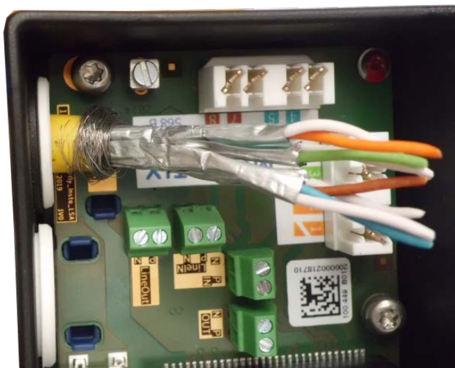
Fig. 23: El cable de red está introducido y el tapón, correctamente colocado
