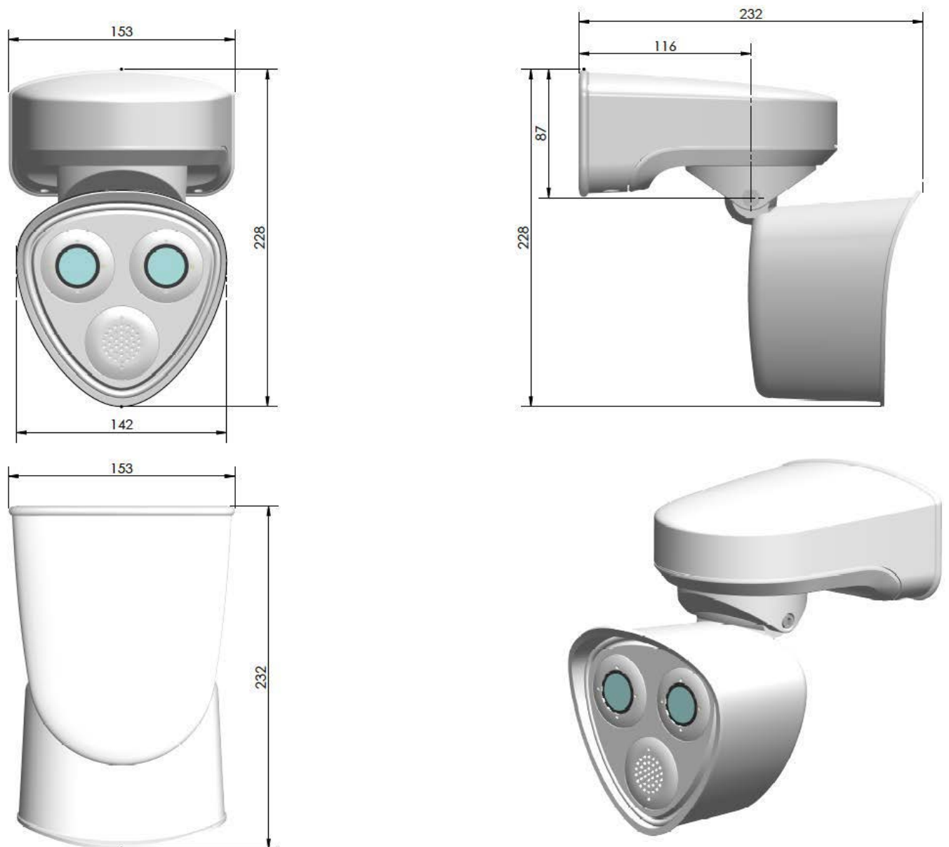
Fig. 4: MOBOTIX M73: Todas las medidas en mm
