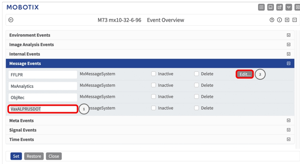
Abb. 26: Beispiel: Generisches Nachrichtenergebnis von Vaxtor USDOT - Number Recognition App
