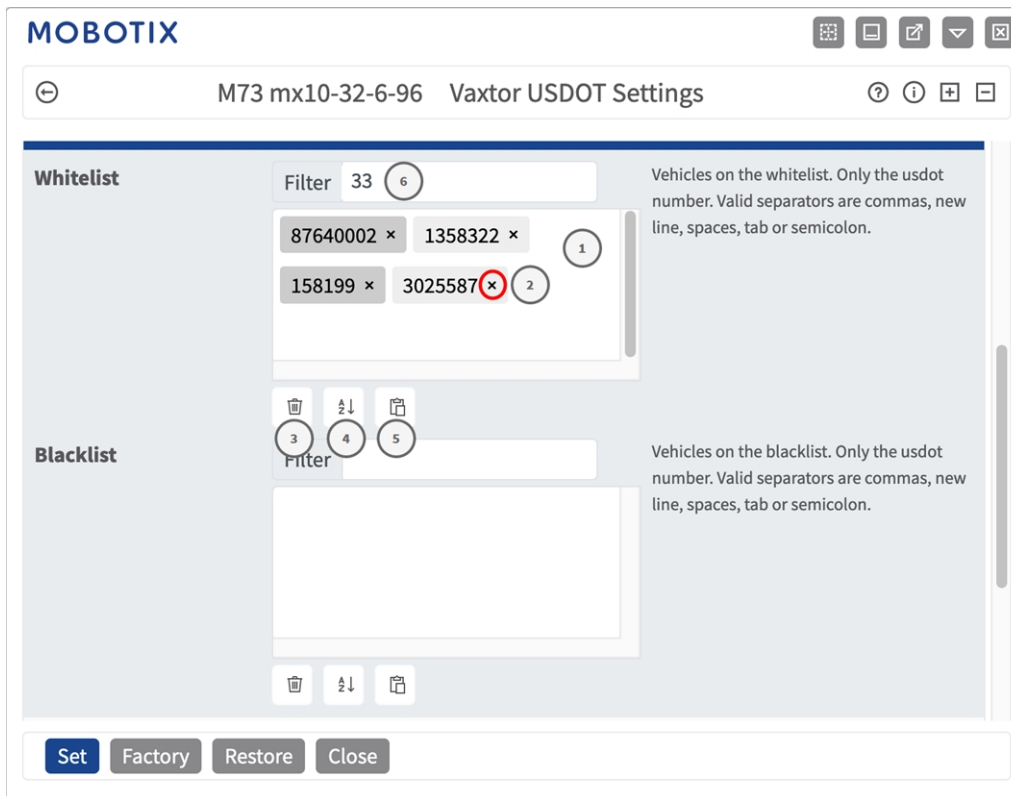
Abb. 15: Schwarze und weiße Liste
