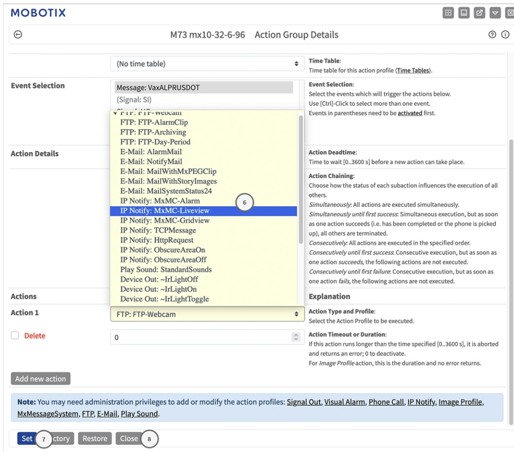
Abb. 22: Aktionstyp und Profil auswählen
