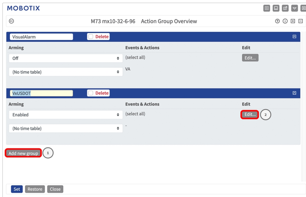
Abb. 20: Definieren von Aktionsgruppen
