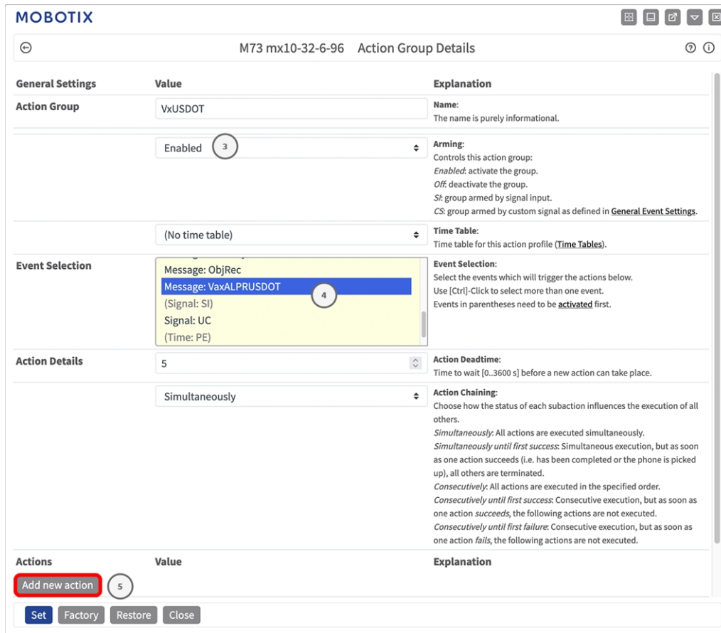
Abb. 21: Konfigurieren einer Aktionsgruppe
