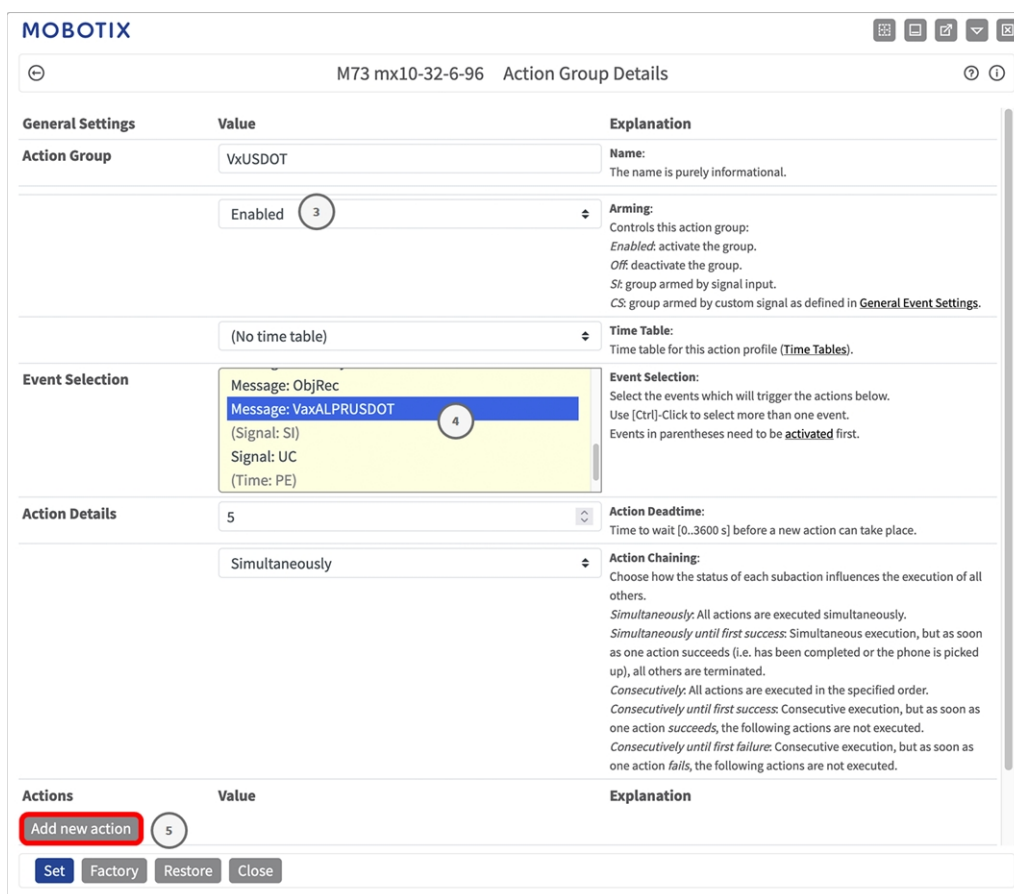
Fig. 22: Configurazione di un gruppo di azioni
