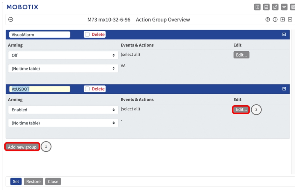
Fig. 21: Definizione dei gruppi di azioni
