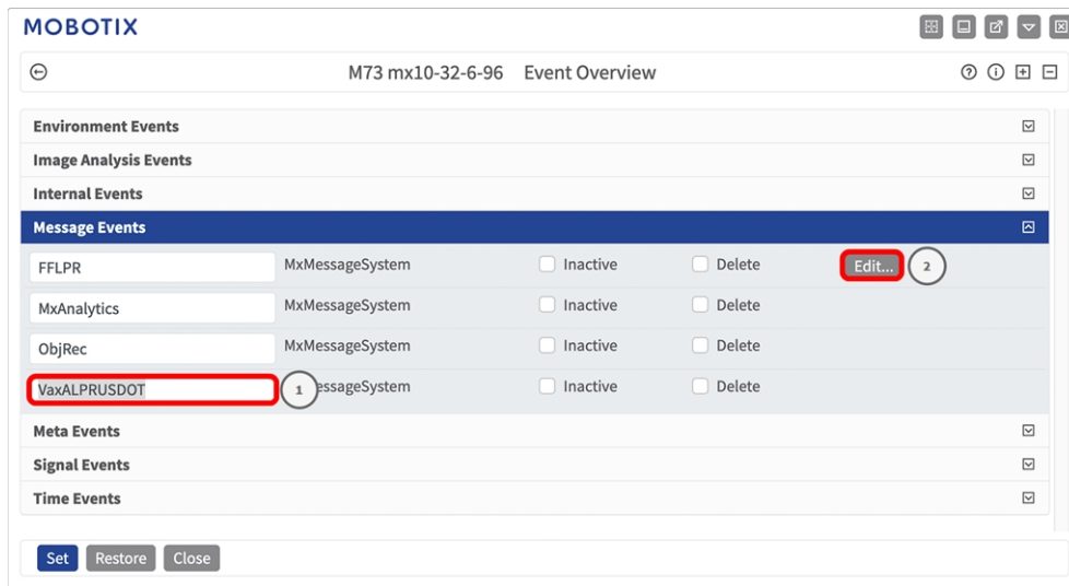
Fig. 27: Esempio: Evento messaggio generico da Vaxtor USDOT - Number Recognition App
