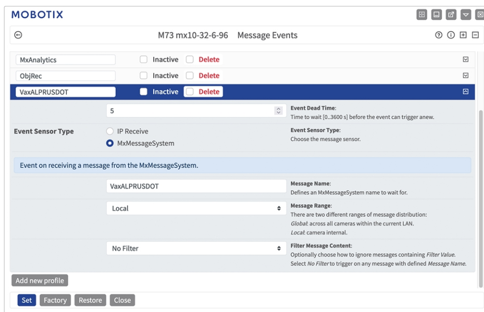
Fig. 20: Esempio: Dettagli evento messaggio generico - senza filtro
