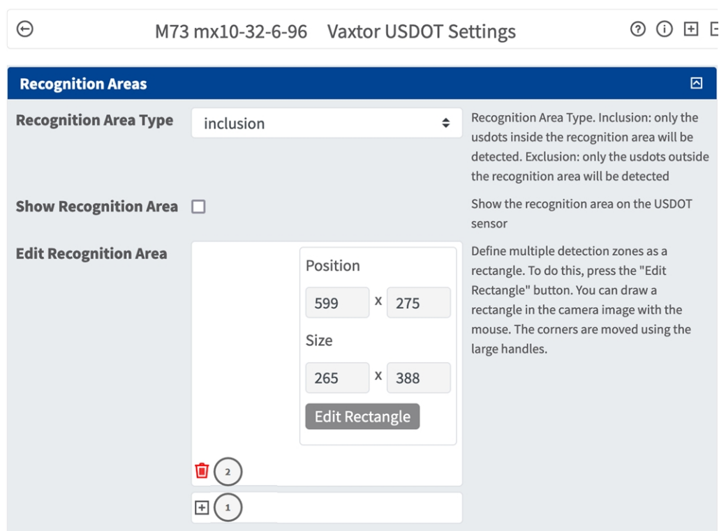
Fig. 15: Scheda "Recognition Areas" (Aree di riconoscimento)
