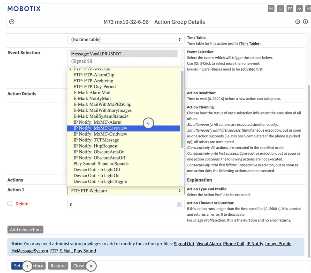
Fig. 23: Selezione del tipo e del profilo dell'azione
