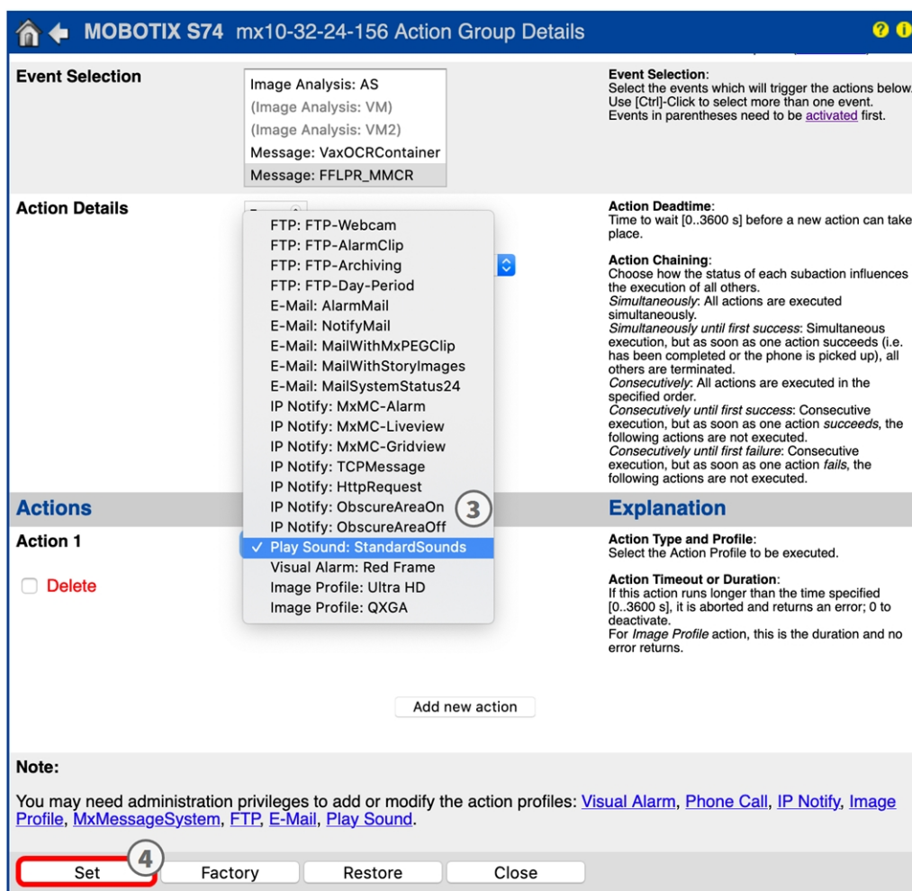
Fig. 24: Selezione del tipo e del profilo dell'azione
