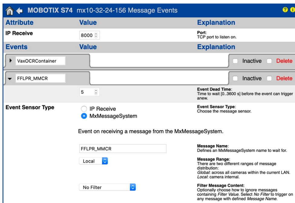
Fig. 21: Esempio: Dettagli evento messaggio generico
