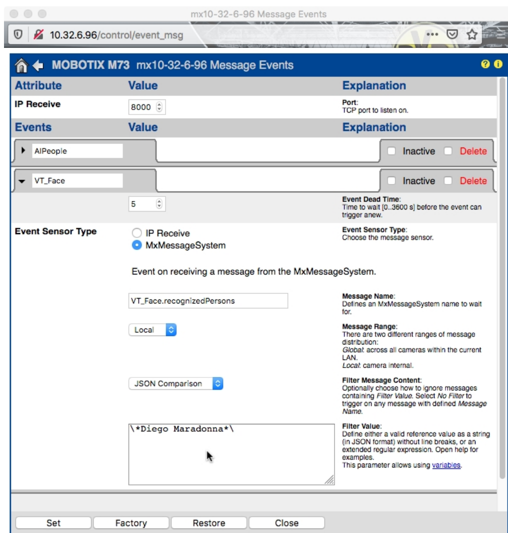
Fig. 27: Configurazione di un evento definito dall'utente
