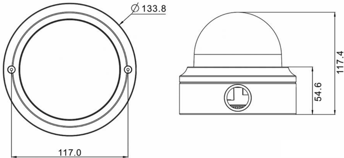
Fig. 1: 2MP Vandal Dome Camera: Todas las medidas en mm
